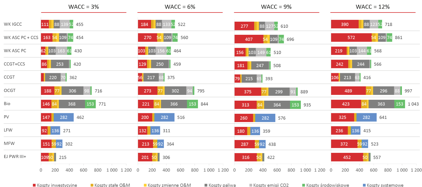
Wykres nr 1. Dekompozycja uśrednionego kosztu całkowitego wytwarzania energii elektrycznej Technologie energetyczne oddawane do eksploatacji w 2035 roku; 30% penetracji technologii OZE w systemie.
