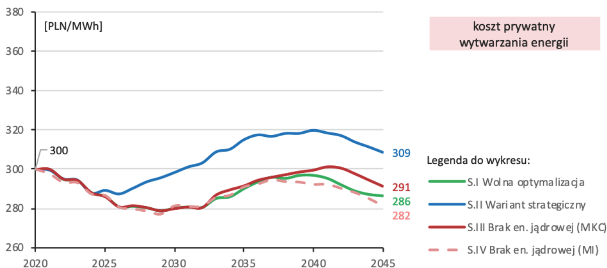
Rysunek 10. Roczny, jednostkowy koszt wytwarzania energii elektrycznej w krajowym systemie elektroenergetycznym (wyłącznie koszt inwestorski) [PLN/MWh]
