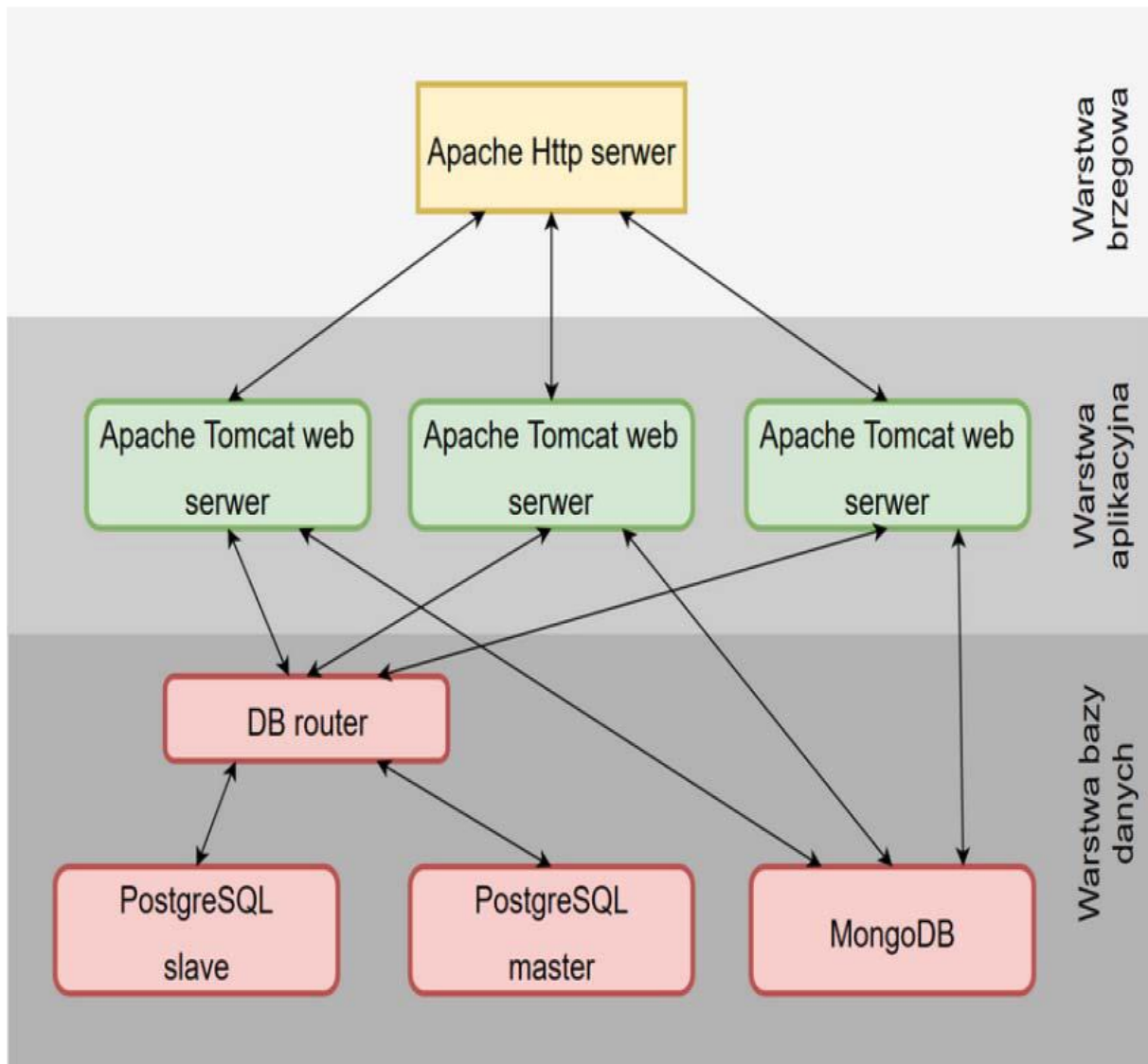
Rys. 1 Schemat komponentów programowych w wielowarstwowej architekturze Rejestru-BDO
