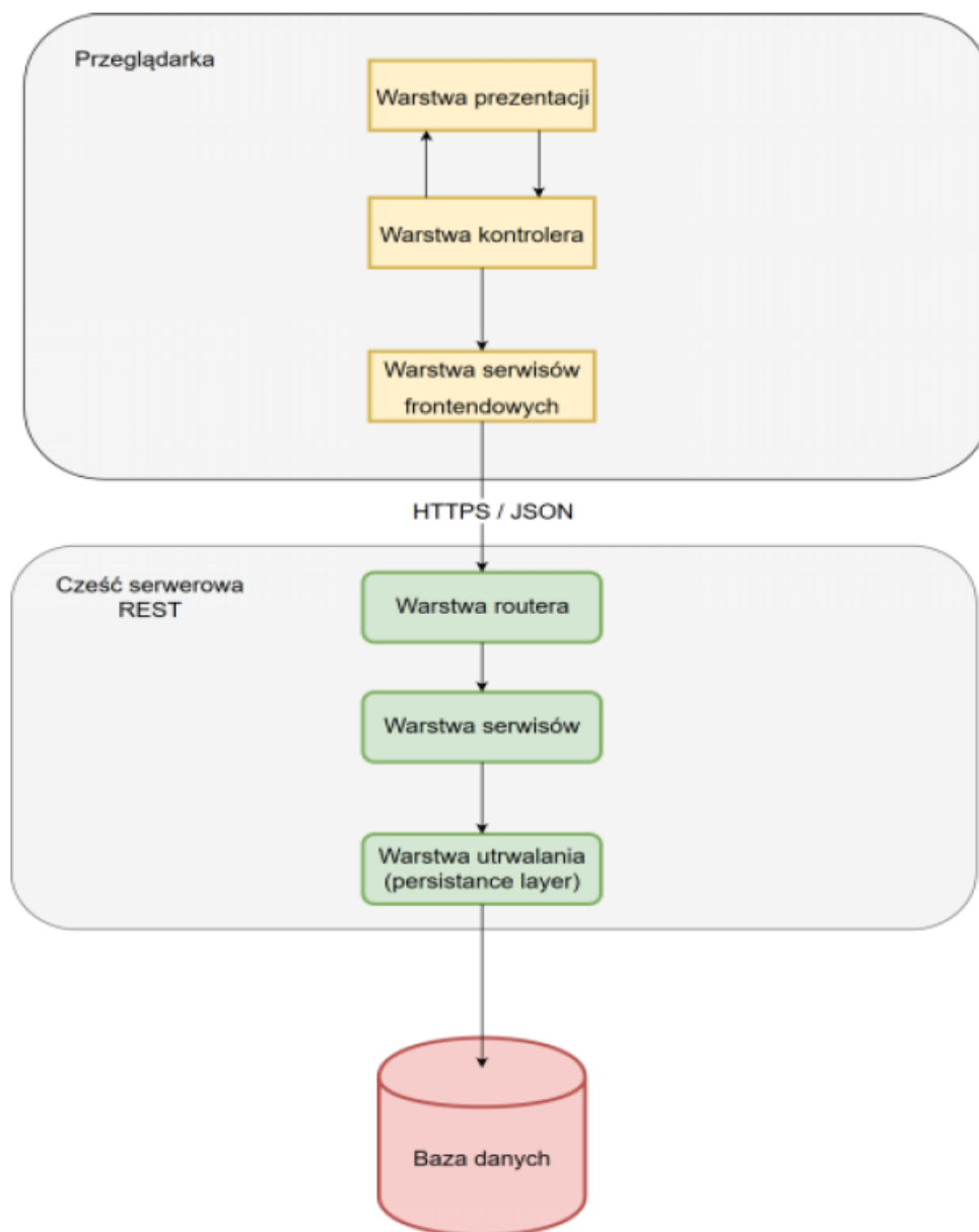
Rys. 2 Schemat architektury aplikacji w wielowarstwowej architekturze Rejestru-BDO
